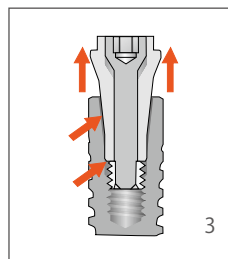
3 固定スクリューを緩めるとプレースメントヘッドがインプラントから離れます。
