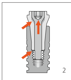
2 プレースメントヘッド内の固定スクリューを緩めます。
