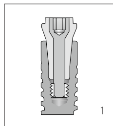
1 インプラントにプレースメントヘッドが固定スクリューによって締められています。
